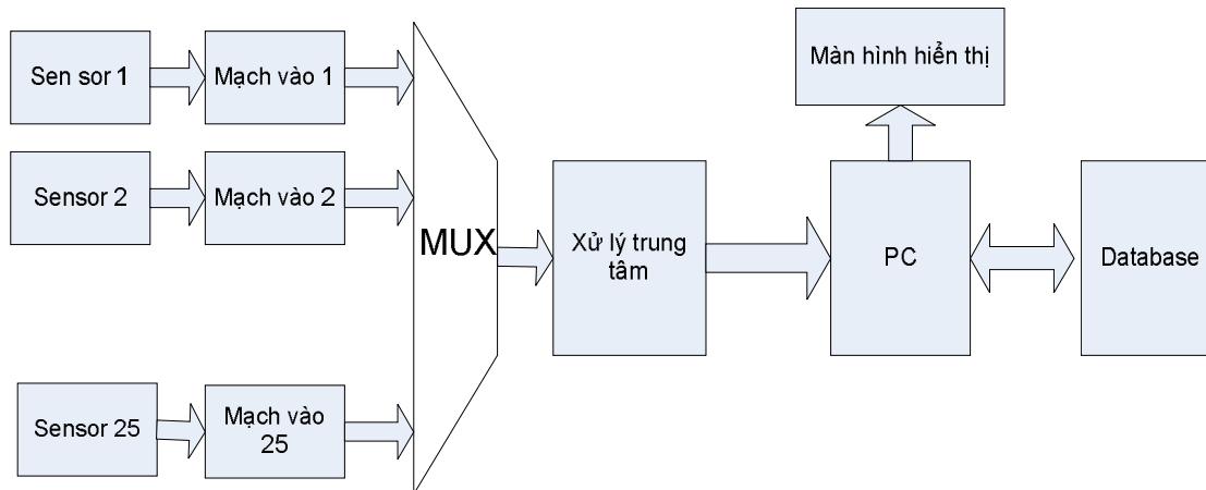
Hình 3. 1. Sơ đồ khối chức năng hệ thống đo nhiệt độ 25 kênh
